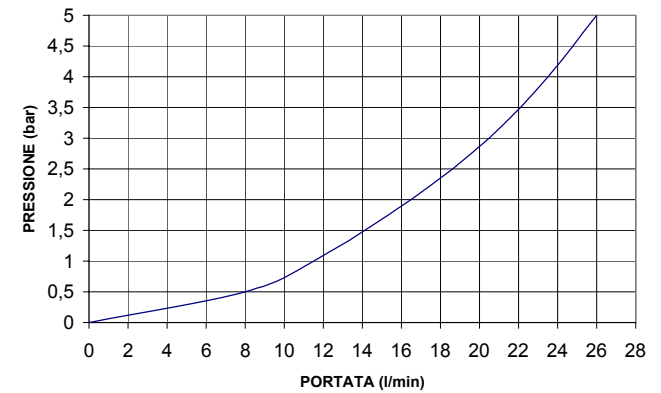
GRAFICO DI PORTATA ART.1215S/1216S
